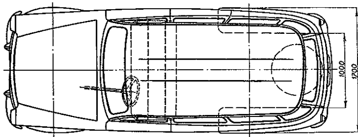
Rozměrový náčrtek dodávkového vozu
