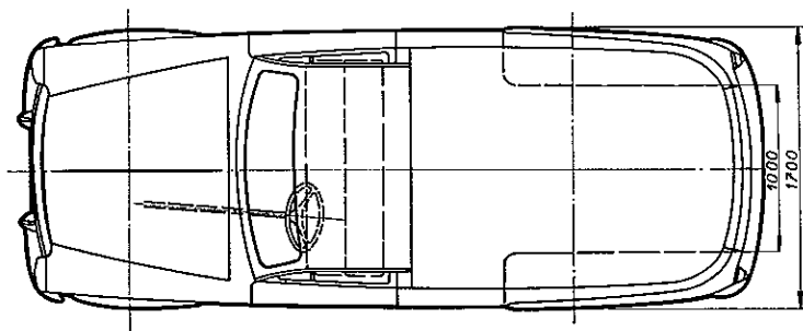
Rozměrový náčrtok vozu PICK-UP
