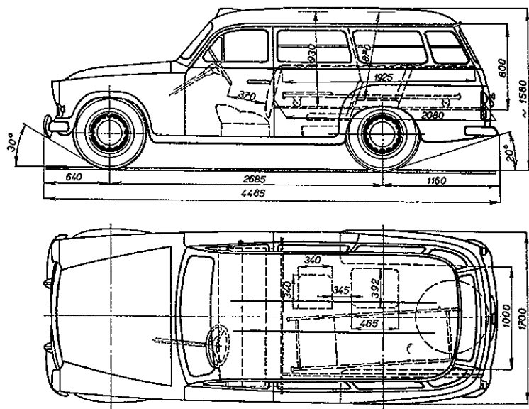
Rozměrový náčrtek zdravotnického vozu
